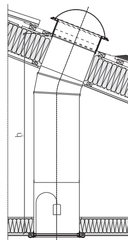
конструкция SFP
