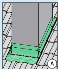
рис.2 (А,Б) – Оклад серии AS
