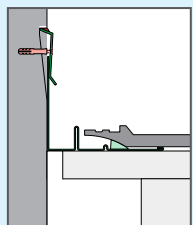
рис.4 – Установка планки примыкания
